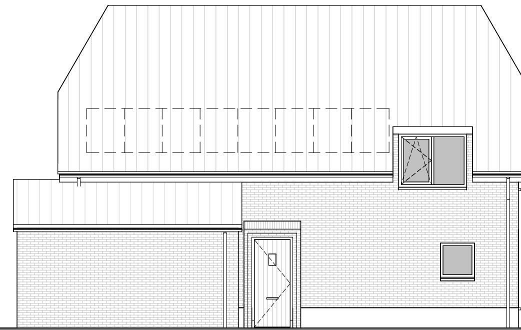
Linkerzijnaanzicht 1:100
