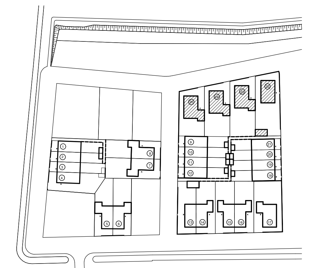
situatie 1:1200
