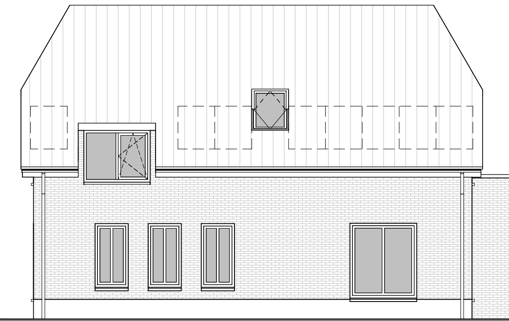
Rechterzijnaanzicht 1:100
