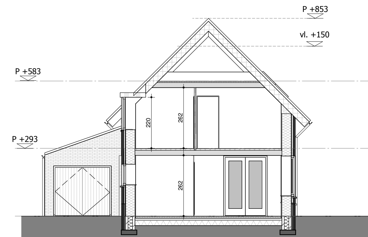
Doorsnede A-A 1:100
