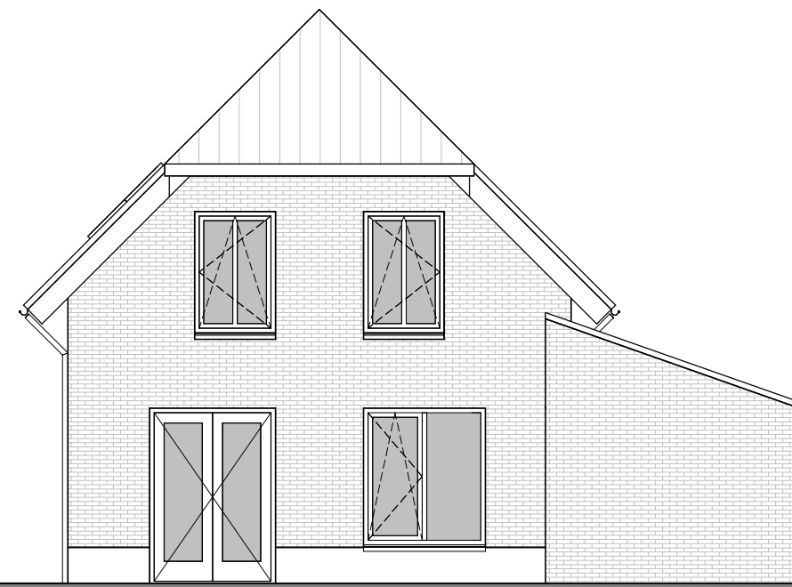
Achteraanzicht 1:100
