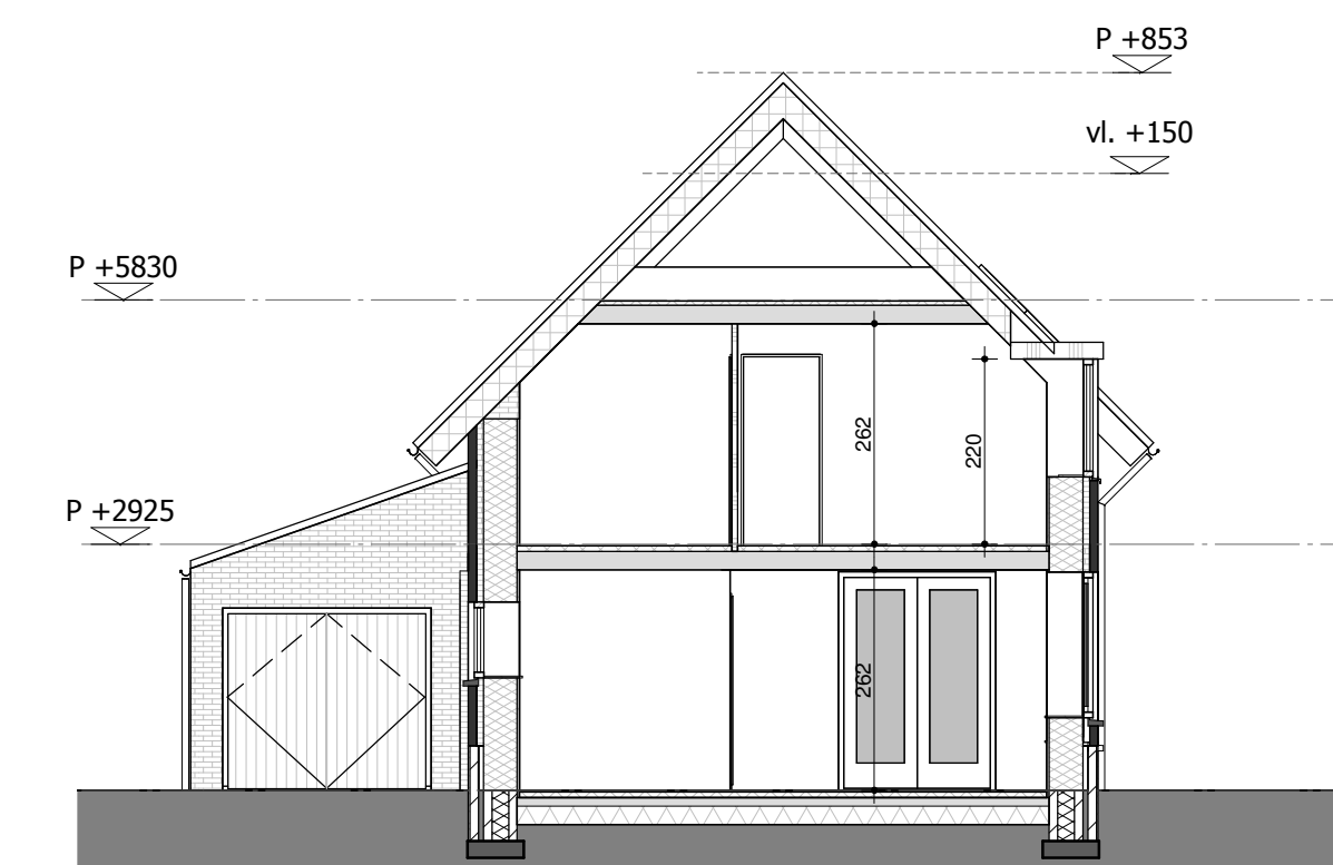
Doorsnede A-A 1:100
