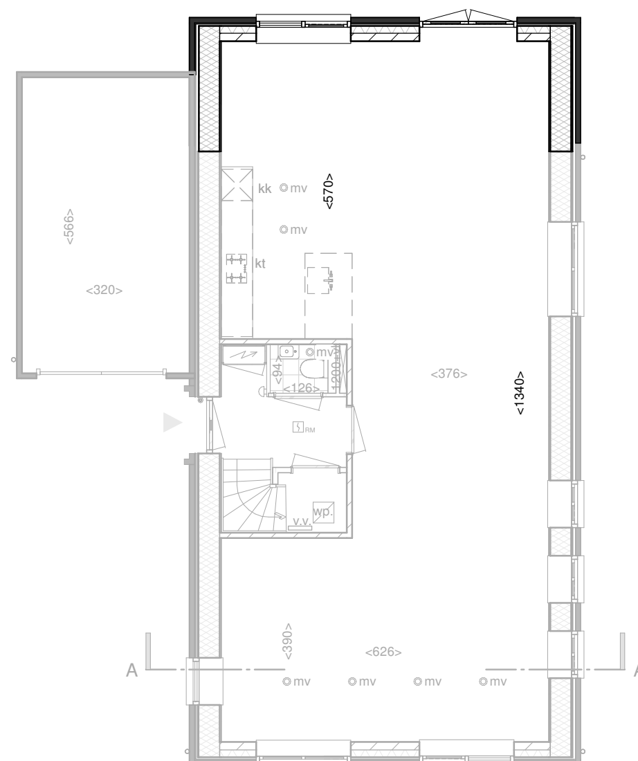
Begane grond 1:100
