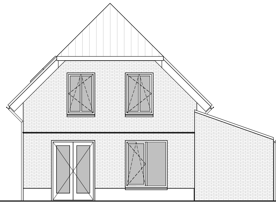
Achteraanzicht 1:100
