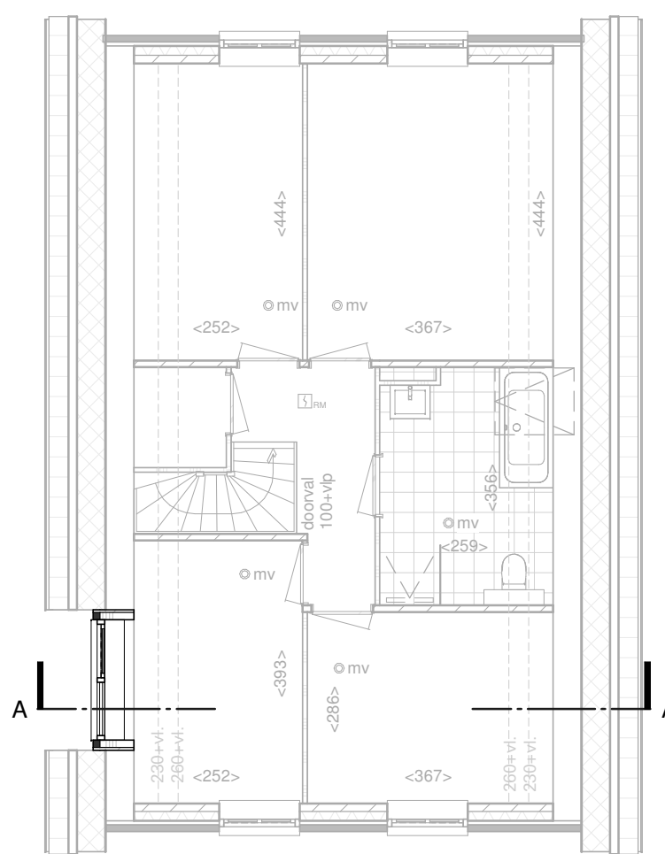
Eerste Verdieping 1:100
