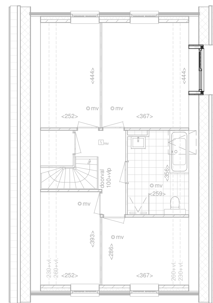
Eerste Verdieping 1:100
