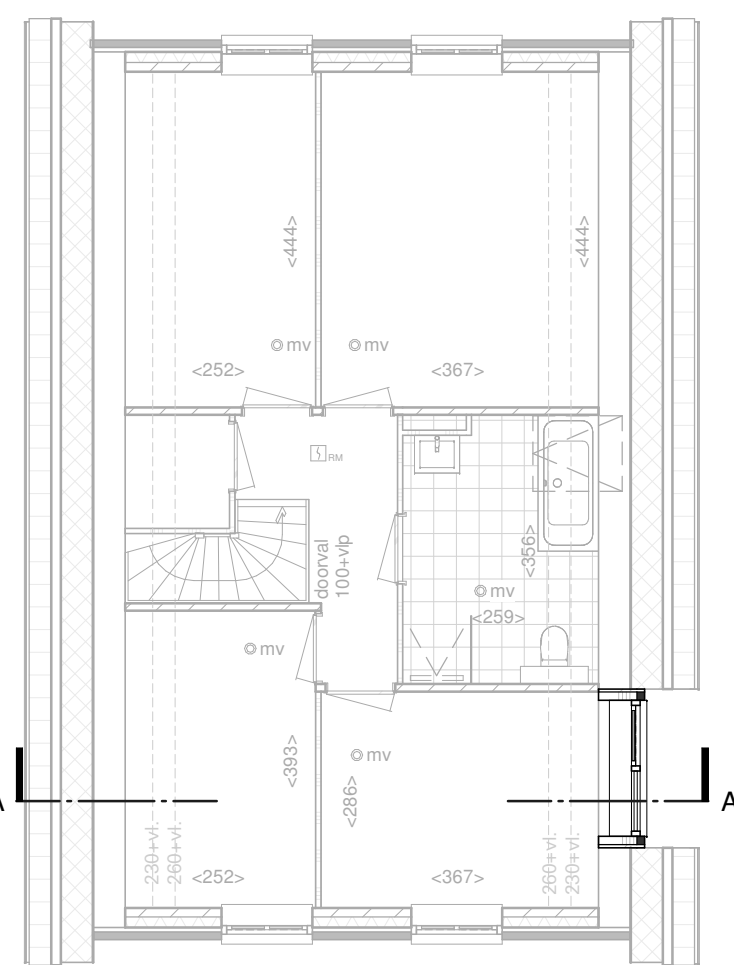
Eerste Verdieping 1:100
