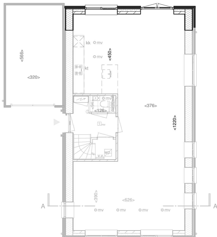
Begane grond 1:100
