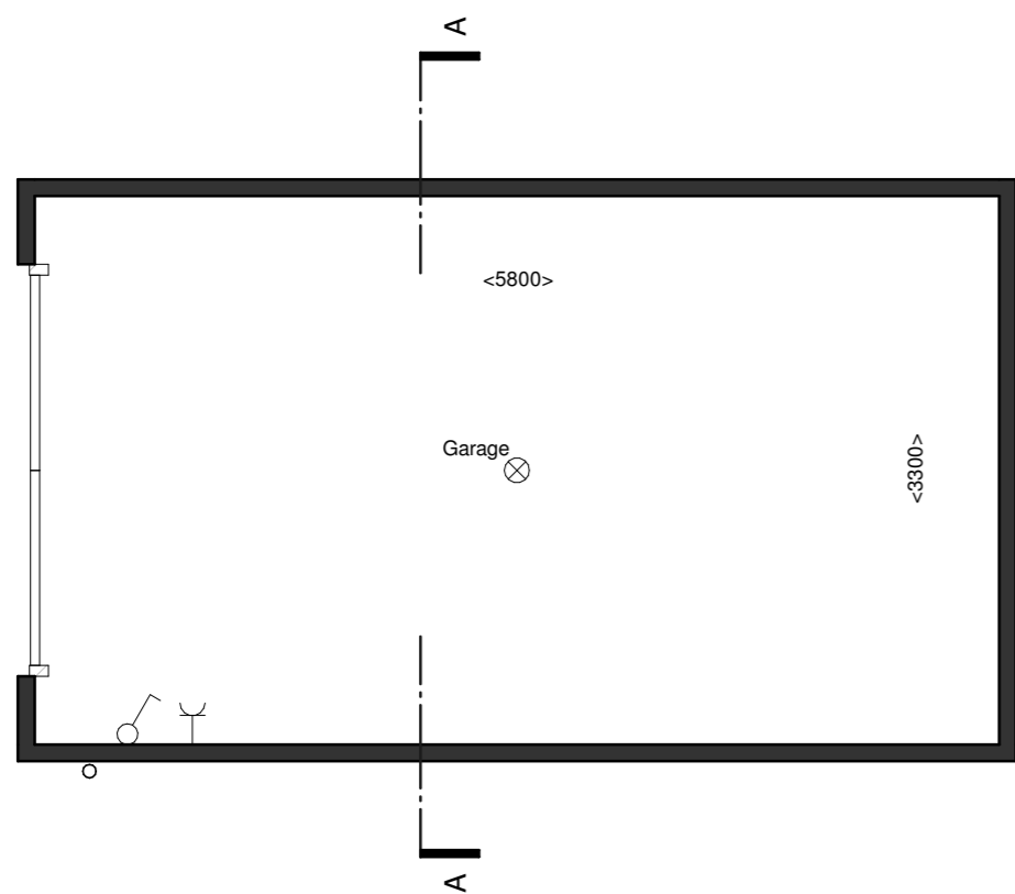
Begane grond 1:50
