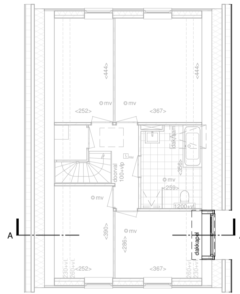
Eerste Verdieping 1:100
