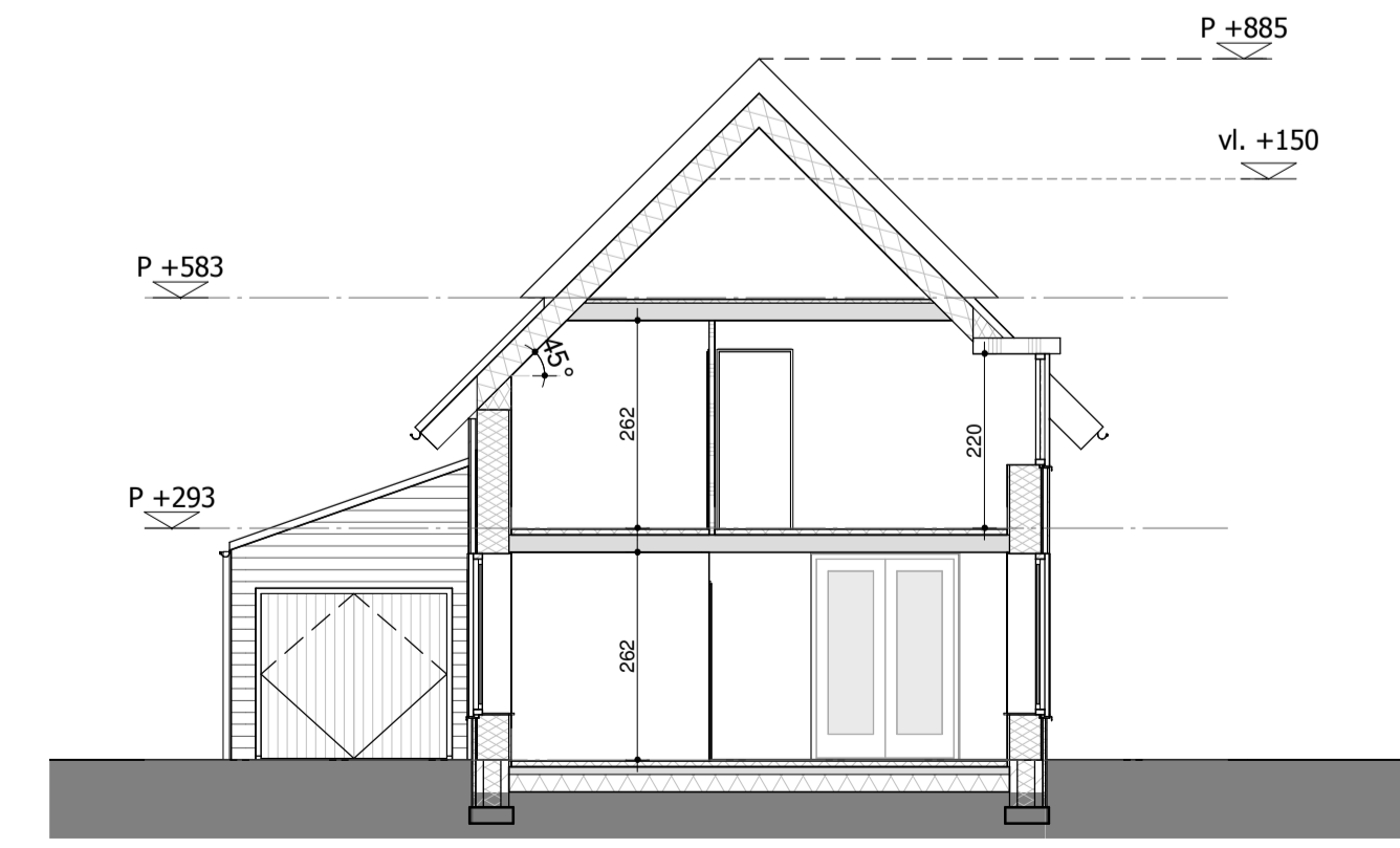
Doorsnede A-A 1:100
