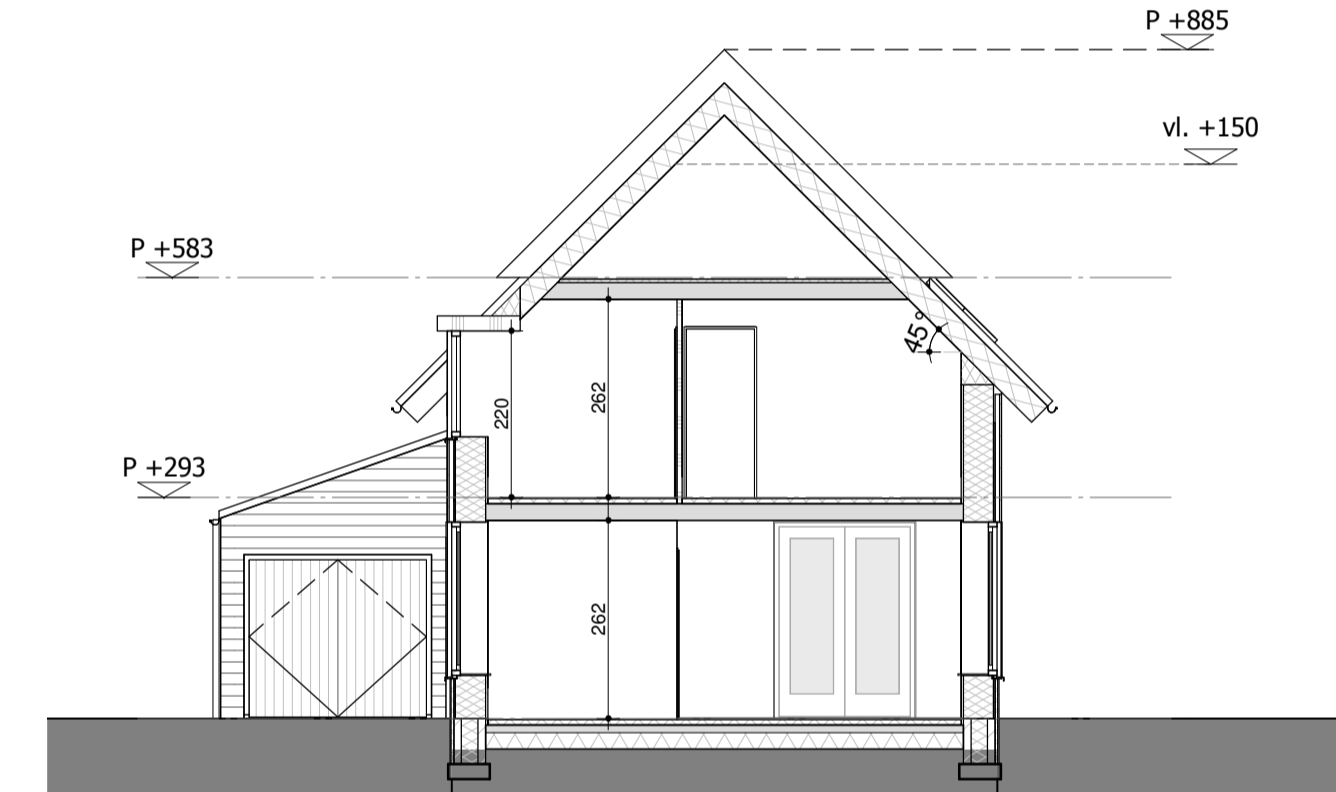
Doorsnede A-A 1:100
