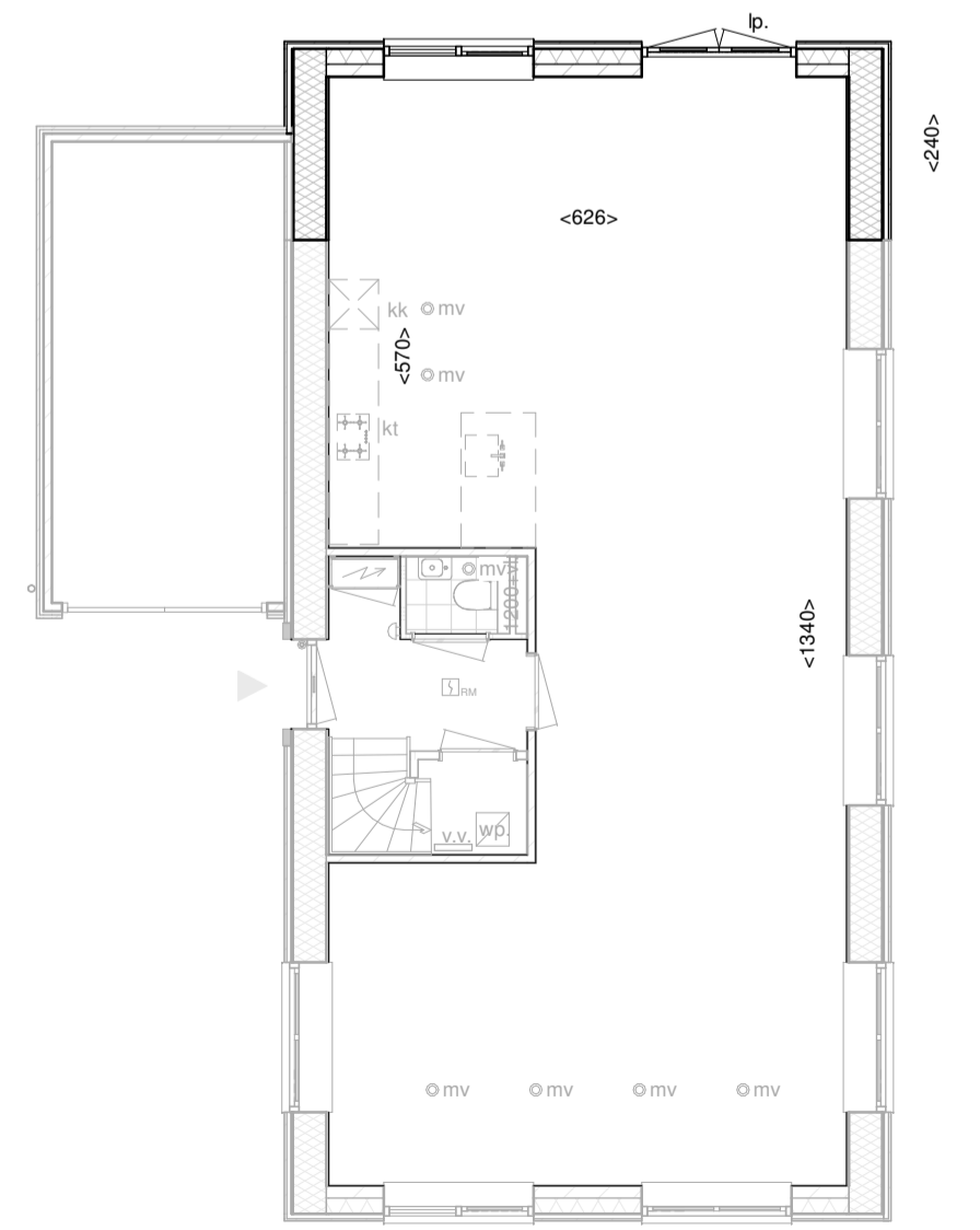
Begane Grond 1:100
