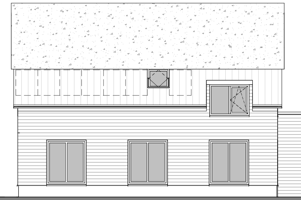
Rechterzijanzicht 1:100
