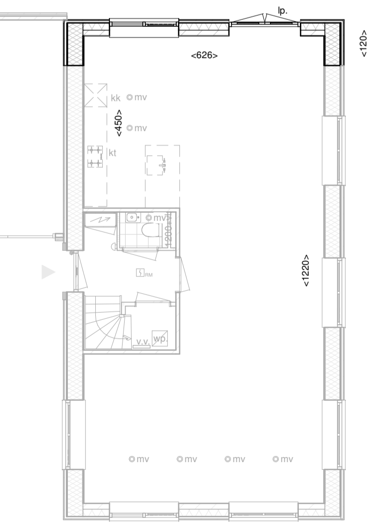
Begane Grond 1:100
